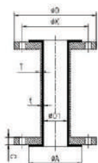
Труба с пластиковым покрытием
