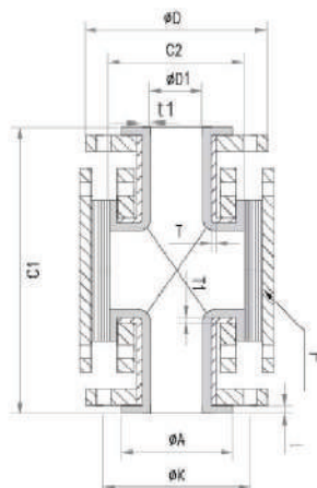
Узел диафрагмы с покрытием PTFE
