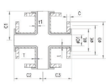
Крестовина с покрытием PTFE
